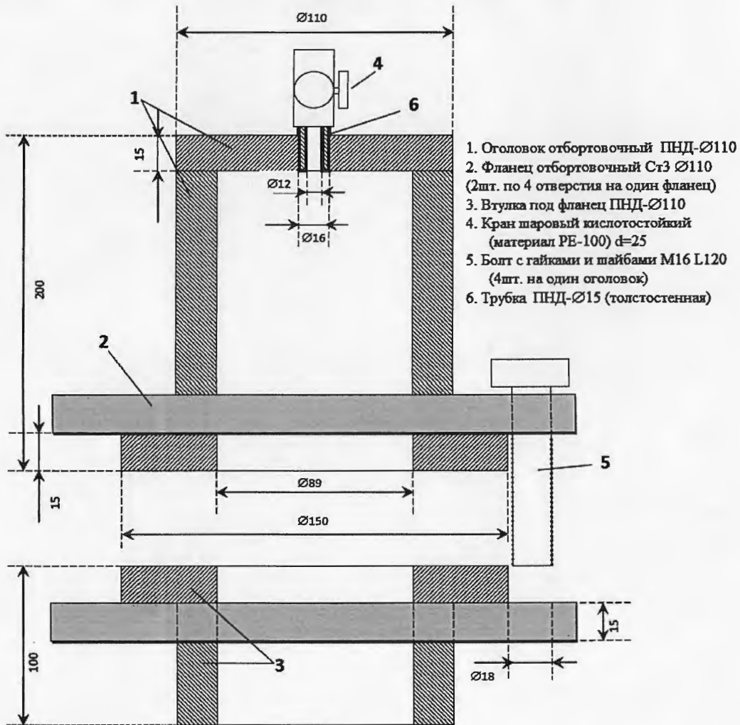
Техническая характеристика №1 Оголовок нагнетательных скважин в комплекте (кислотостойкий) Ру-8 бар
